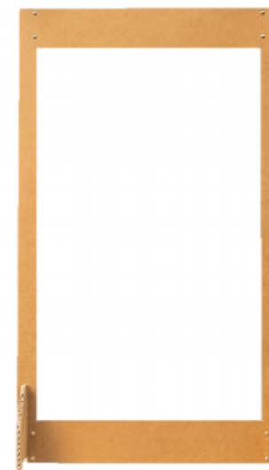
Dimensioni esterne:1000x1800 mm Dimensioni foro 1480x860 mm
